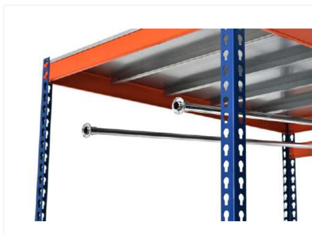
37 Берем трубу (штанги) и одним концом вставляем в установленный фланец на стяжке, а на второй конец трубы устанавливаем второй фланец.
